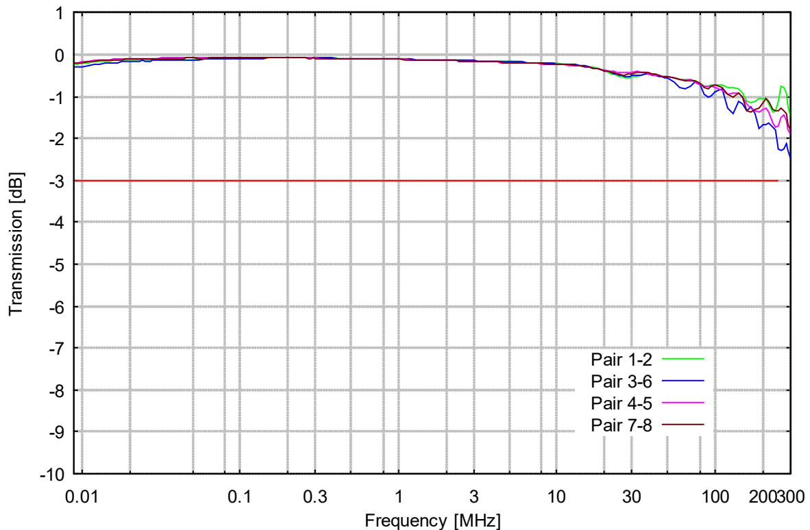
Bild 4: typ. Transmission AE-EuT (symmetrisch) Fig. 4: typ. Transmission AE-Eut (differential mode)
